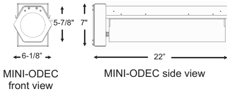
Mini ODEC with Pan/Tilt Link to data sheet
